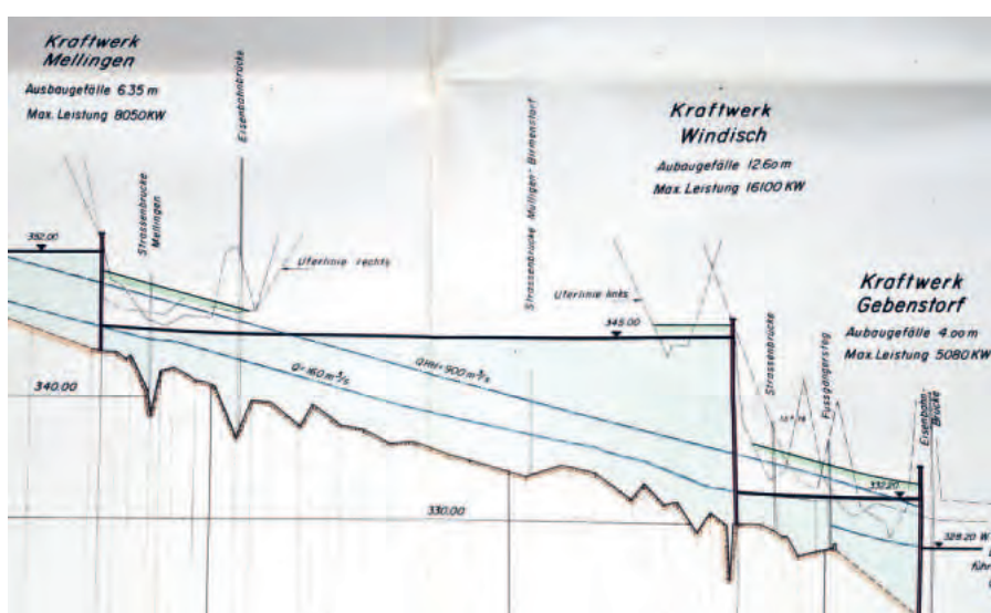
Längsprofil der Kraftwerkstufen Mellingen, Windisch und Gebenstorf (beide Abbildungen aus Wasserwirtschaftsplan der Reuss 1959, Motor Columbus AG)
